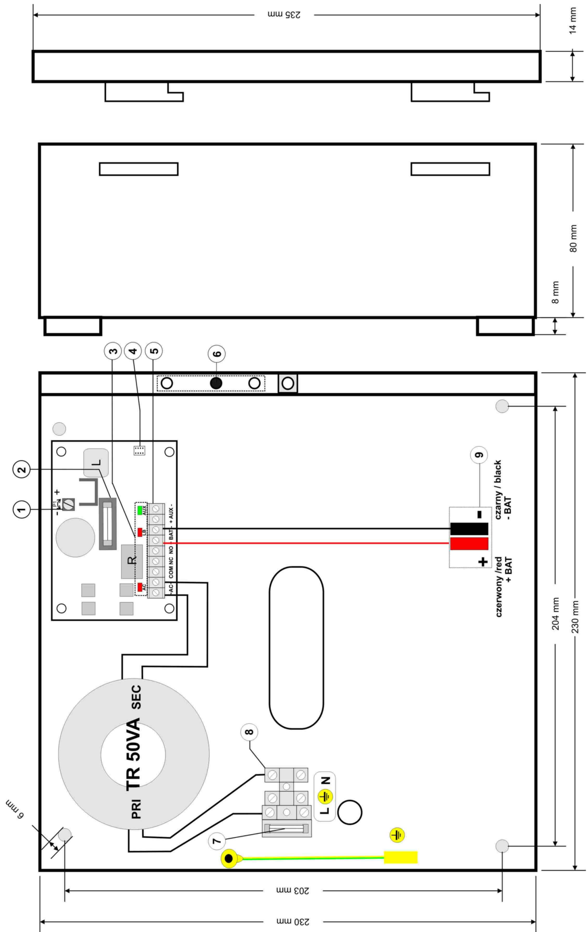
Rys.2. Widok zasilacza.
