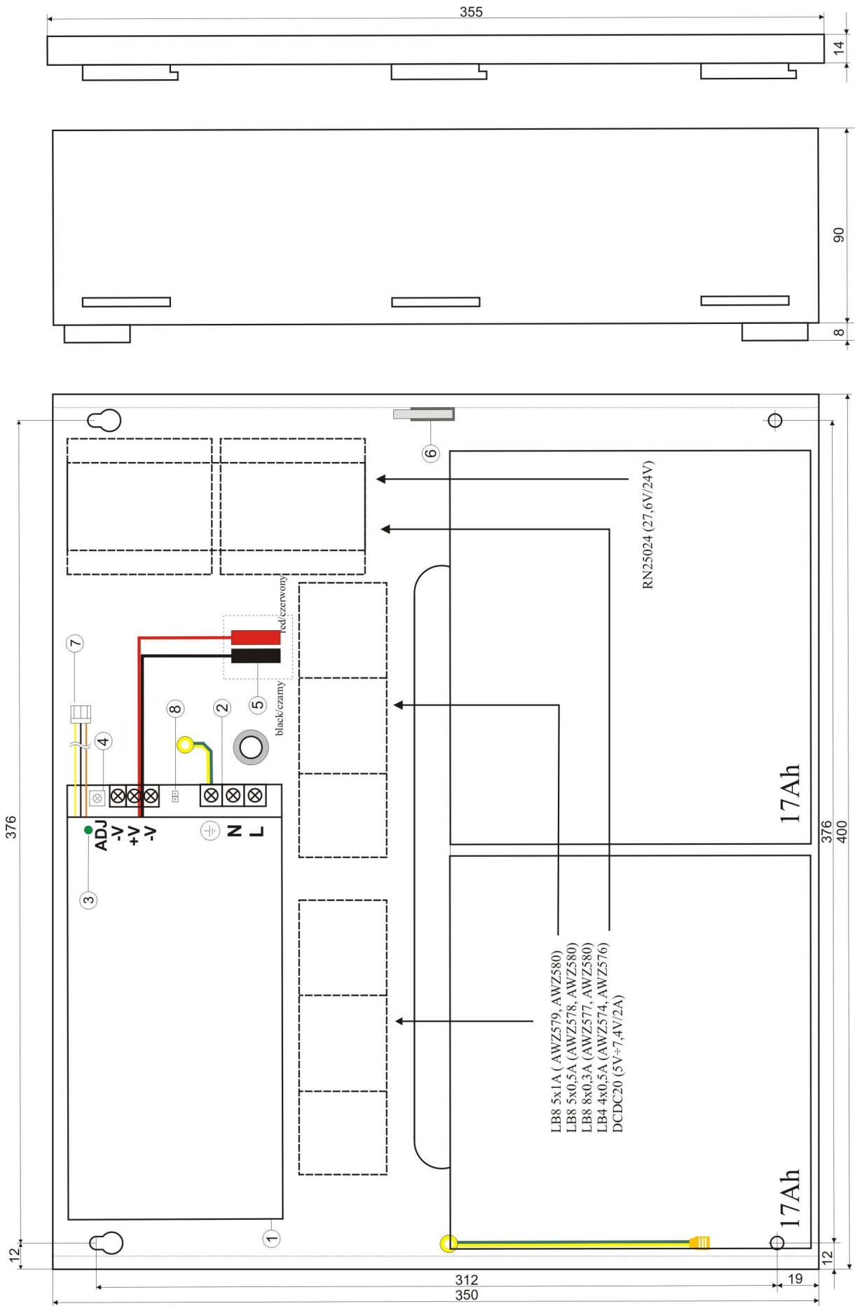
Rys.2. Widok zasilacza.
