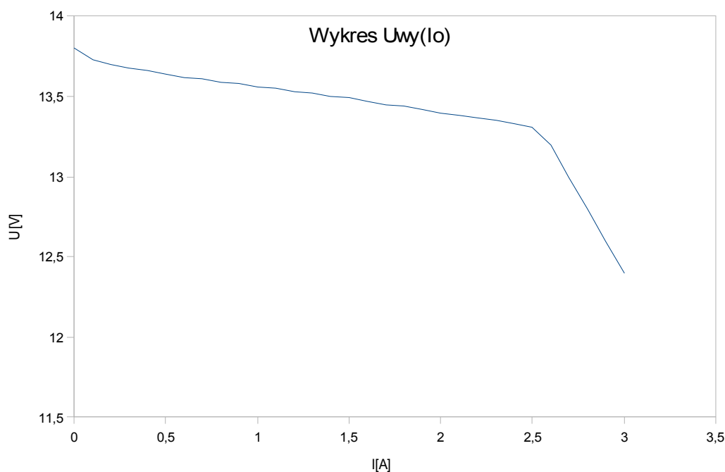
Rys.3. U_{wy}=f(I_o)
