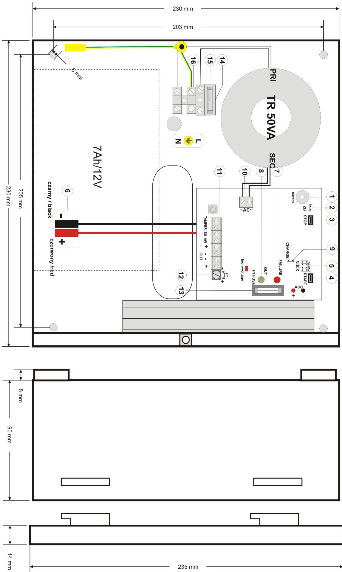
Rys.2. Widok zasilacza
