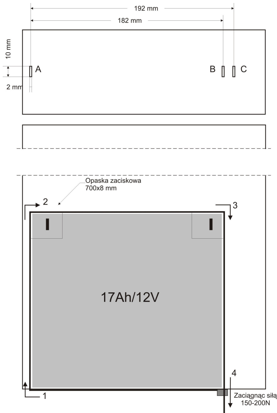
Rys.4. Procedura mocowania akumulatora.
