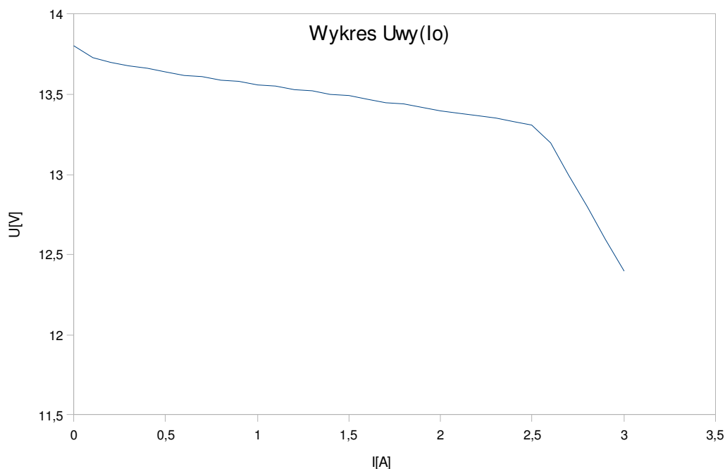
Rys.3. U_{wy}=f(I_o)
