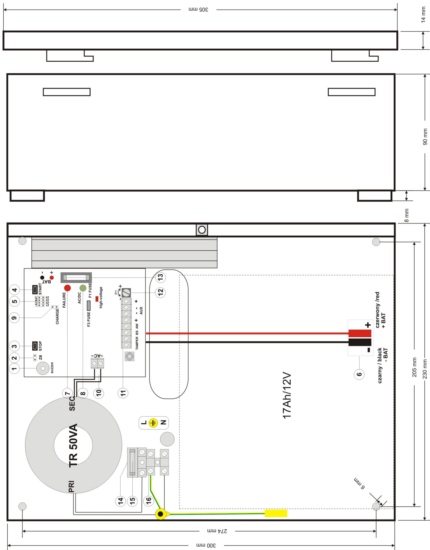
Rys.2. Widok zasilacza.
